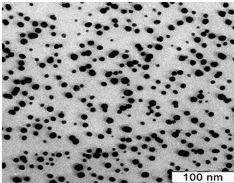
Рис. 2. Электронная микрофотография наночастиц серебра
