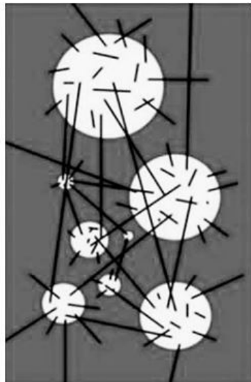
Рис. 3. Модели Большой Вселенной – без тоннелей (слева) и с тоннелями (справа). Так представляют топологию «кратовых нор» акад. Н.С.Кардашев и его коллеги [3–4]
