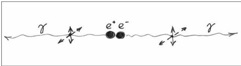
Рис. 6. Эффект Эйнштейна – Подольского – Розена
