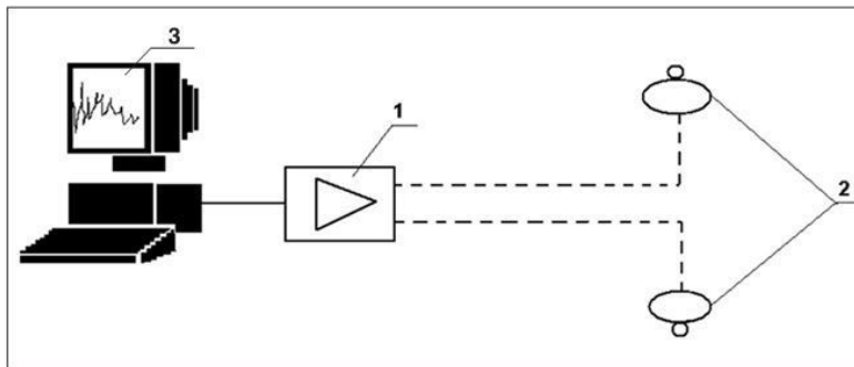
Рис. 1. Структурная схема измерительного комплекса «Эниотрон-3»
