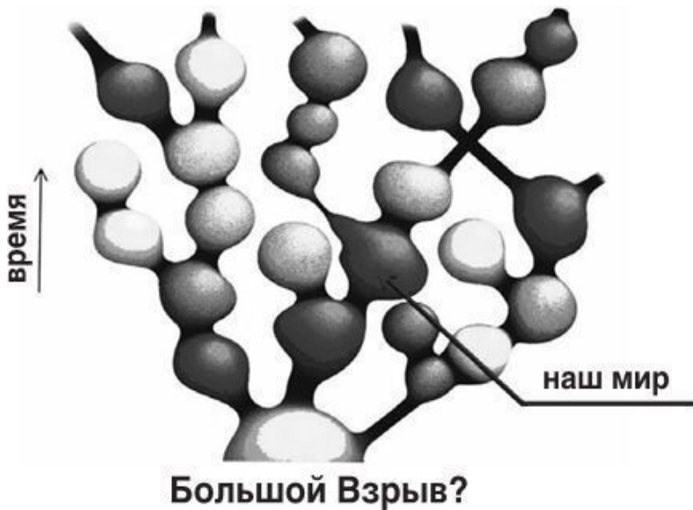
Рис. 6. Мультиверс (по А.Линде)
