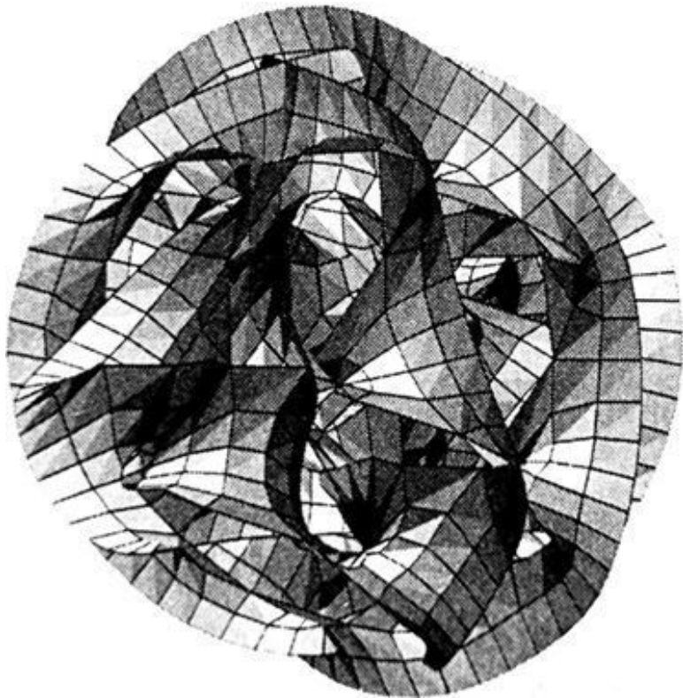
Рис. 5. Дополнительные (свернутые) пространственные измерения в теории суперструн (по Б.Грину [14, с. 142])
