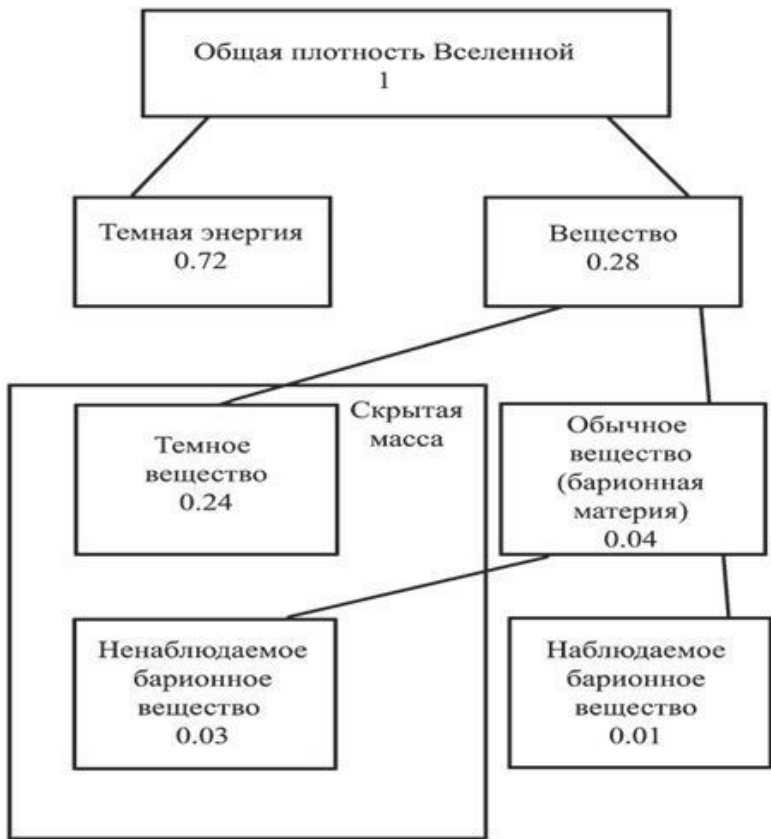
Рис. 3. Доля различных видов материи во Вселенной («Земля и Вселенная», 2006. № 5. С. 49)
