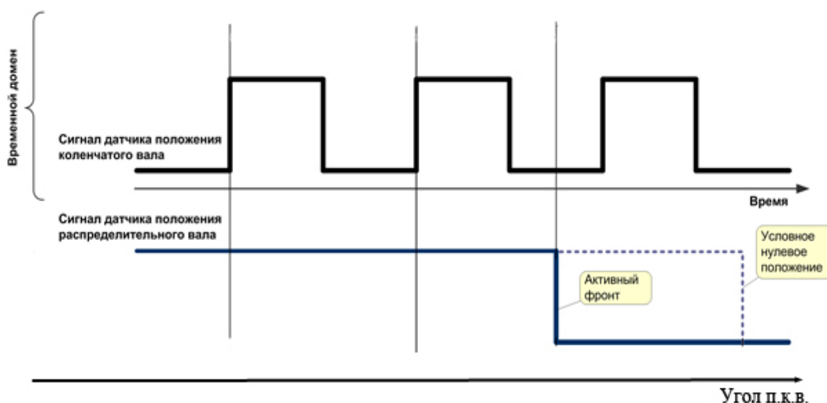
Рис. 2.20. Диаграмма синхронизации коленчатого и распределительного вала ДВС автомобиля с КЭУ
