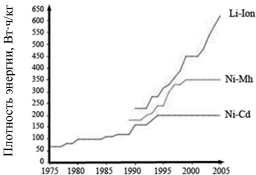
Рис. 1.9. Исторические достижения в области повышения энергоэффективности ТАБ
