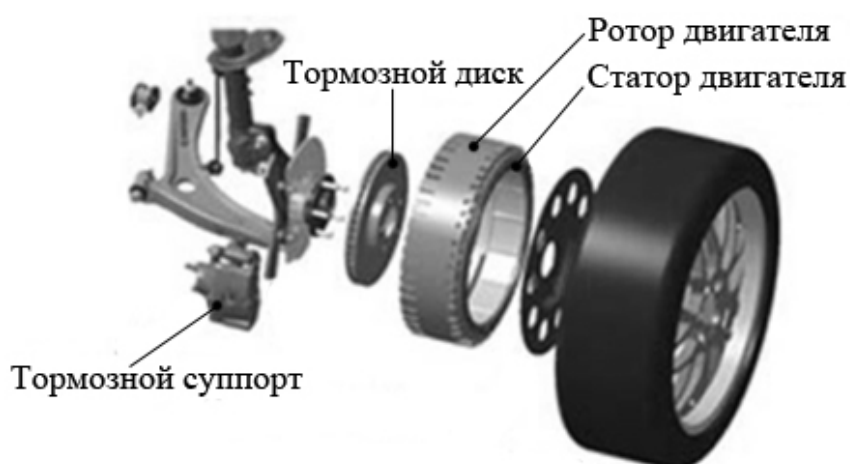
Рис. 1.14. Конструкция электропривода колес Mitsubishi
